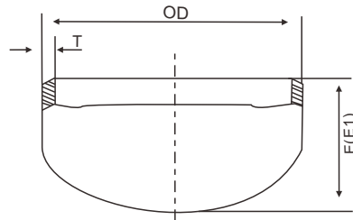
Pipe cap
